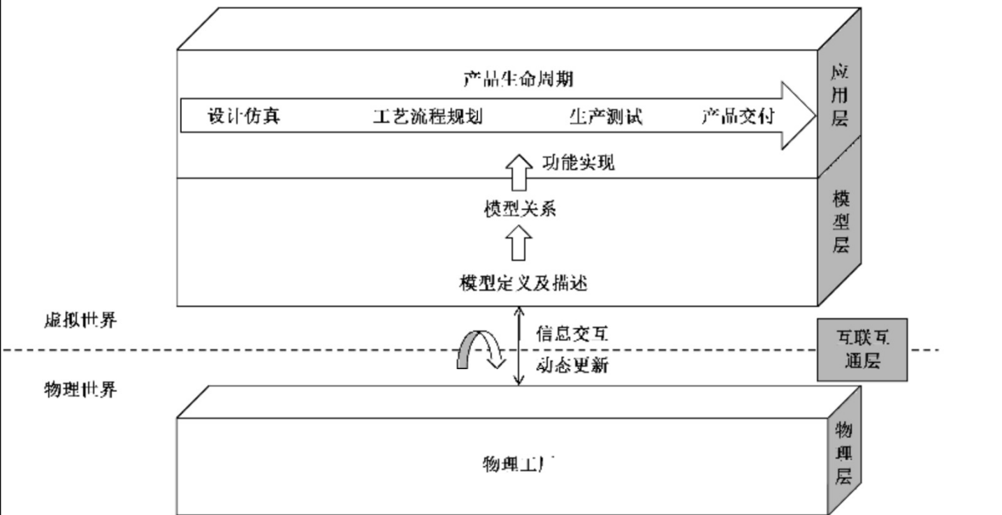
图 1 虚拟工厂参考架构
